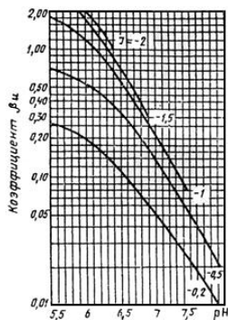
Рис.4. Номограмма для определения коэффициента \beta_k при расчете дозы щелочи
