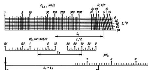
Рис.1. Номограмма для определения pH насыщения воды карбонатом кальция ( \text{pH}_s )
