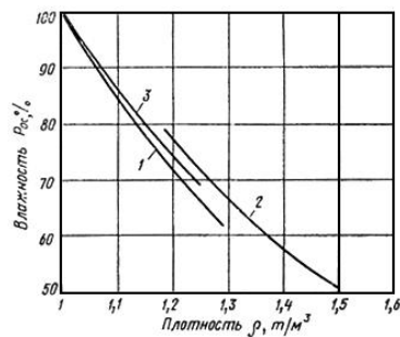
Рис.6. Значения плотности в зависимости от влажности осадка станций обезжелезивания и реагентного умягчения воды
