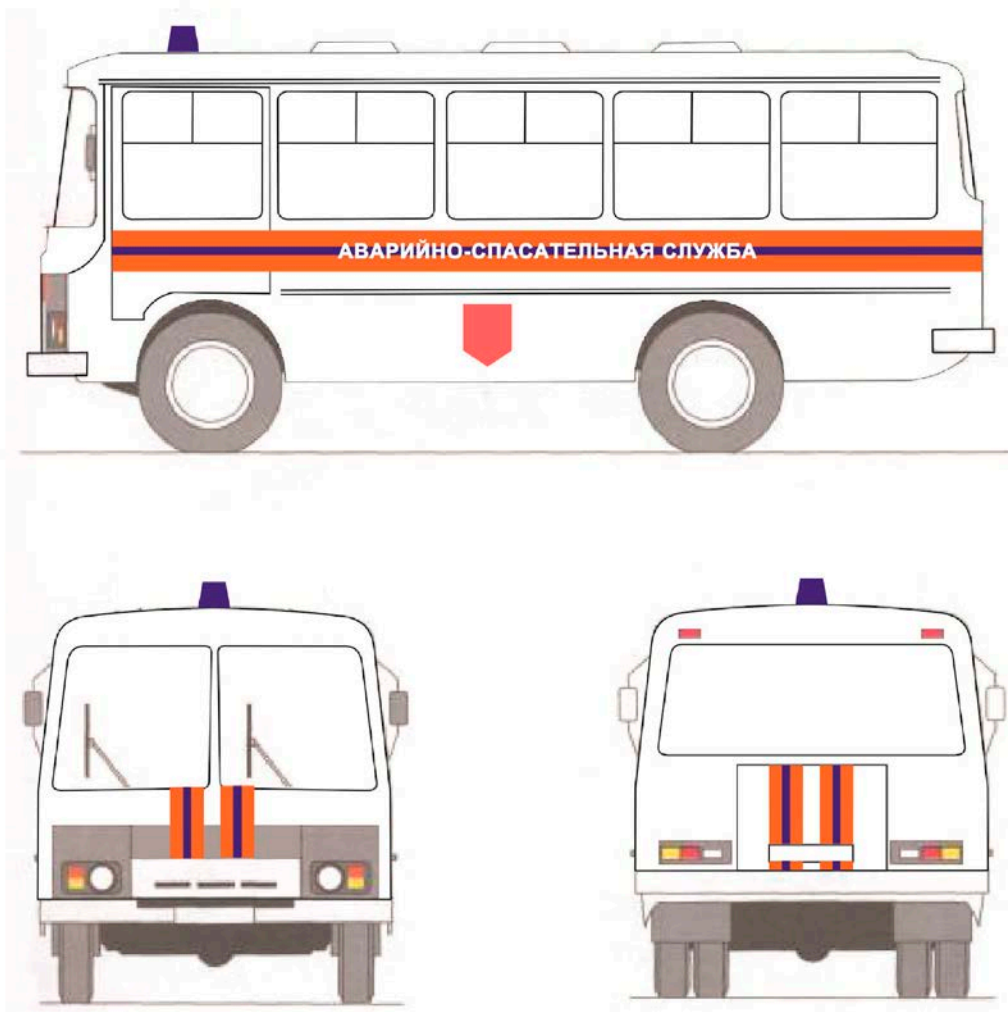
Рисунок А.5 - Цветографические схемы автомобилей Министерства по делам гражданской обороны, чрезвычайным ситуациям и ликвидации последствий стихийных бедствий ДНР
