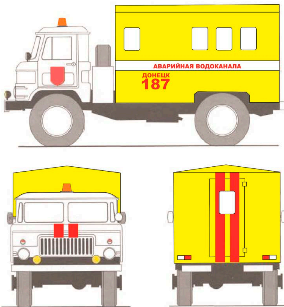
Рисунок А.27 - Цветографические схемы автомобилей аварийных служб Министерства строительства и жилищно-коммунального хозяйства ДНР
